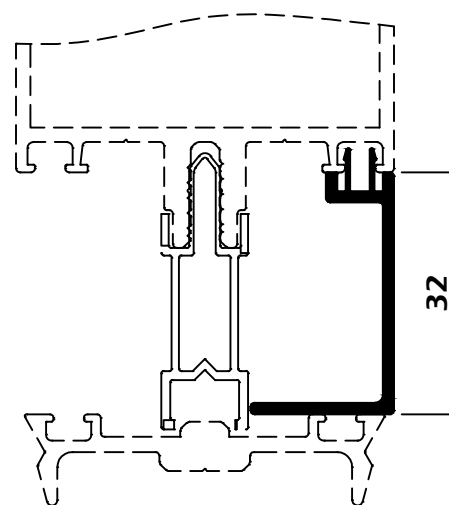
ext FC50.35 Perfil de fecho Travessa de 24mm
