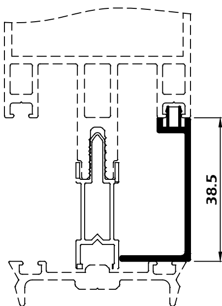
ext FC50.36 Perfil de fecho Colume de 24mm
