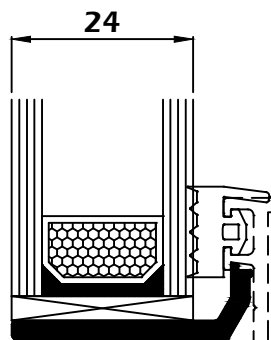
ext FC50.37 Suporte de vidro de 24mm.
